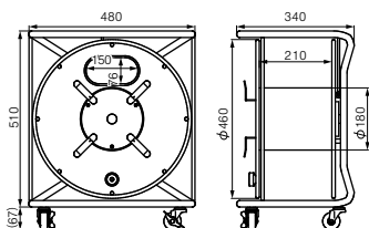
R460-S
