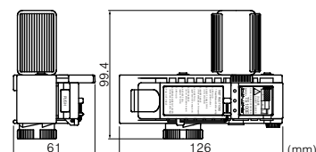
TS100E
