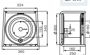
R300
