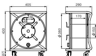
R380-S
