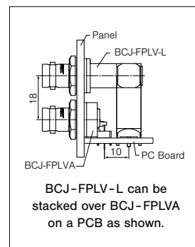
BCJ-FPLV-L
