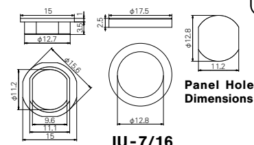
IU-7/16
