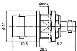
BCJ-HBCJK
