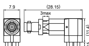
HBCJ-LRK/1
