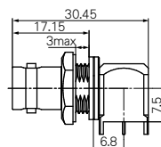
BCJ-FPLV-12G
