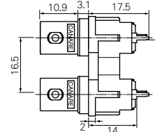
BCJ-BPC2P
