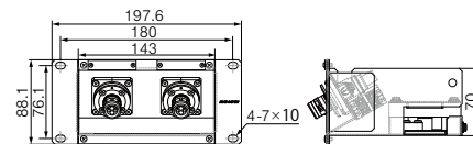
COPS-FF2A
