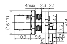
BCJ-FPLV01
